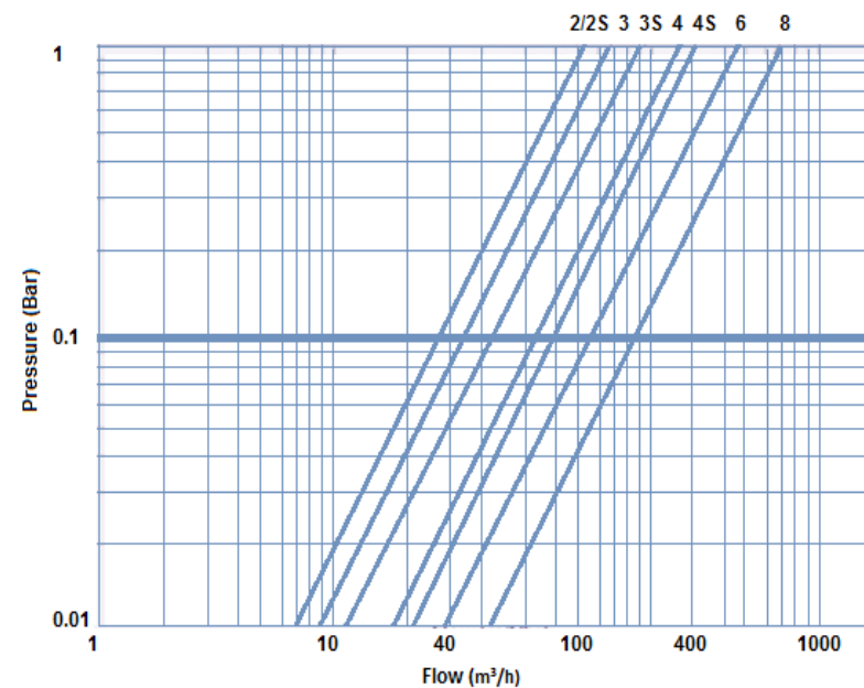
Потеря давления при 120 микрон
