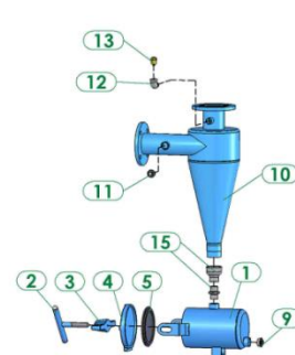
Модель F710-F755
