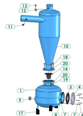
Модель F760
