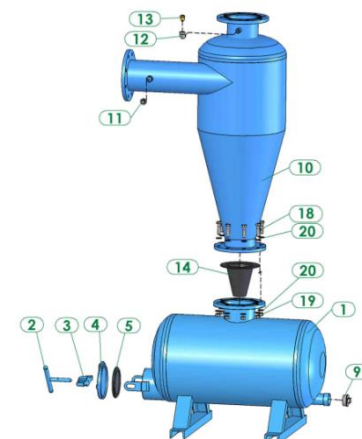
Модель F770-F780
